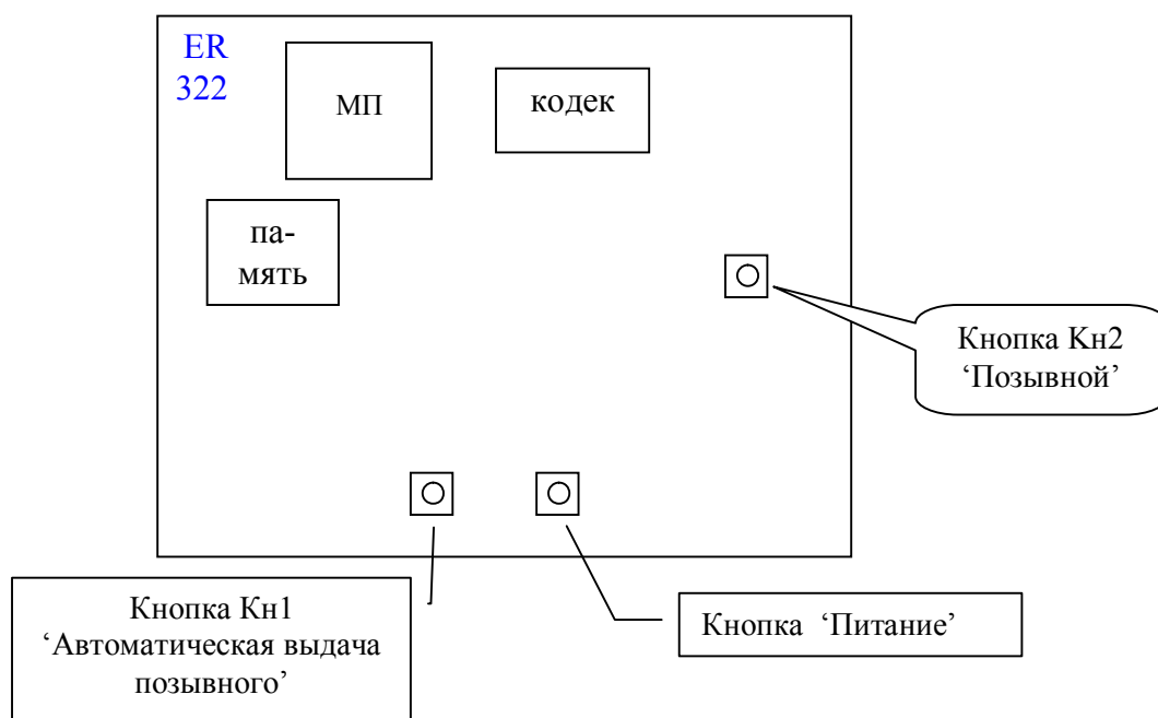
Рис. 2. Вид на печатную плату репитера
